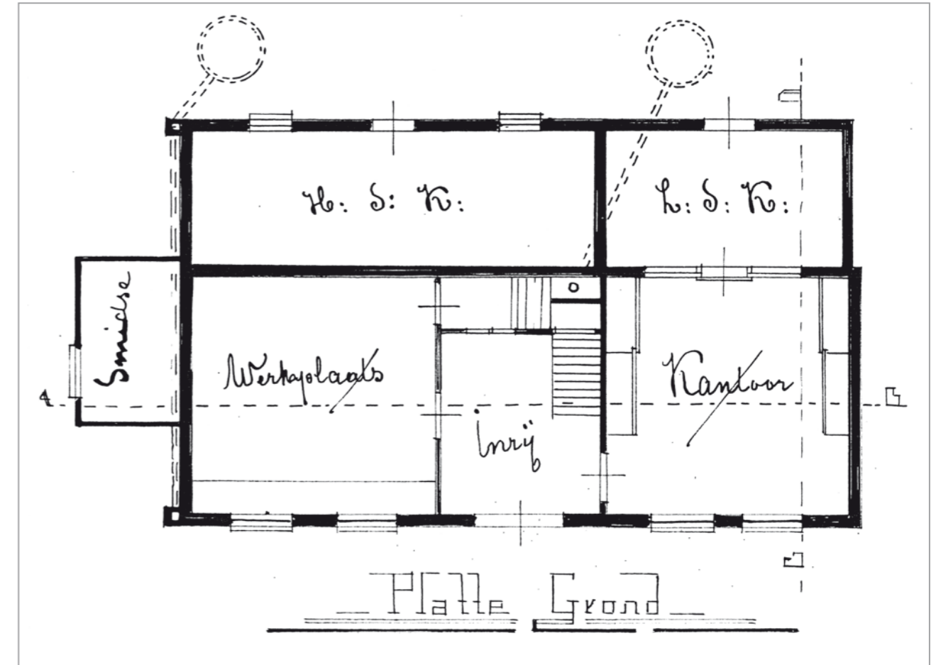
Weer de bouwtekening van 1913. De letters H:S:K en L:S:K betekenen vermoedelijk Hoge Stroom Kast en Lage Stroom Kast.
